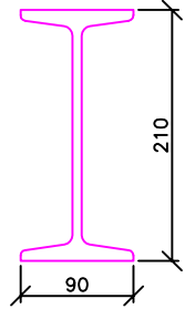
9 - podélný profil
