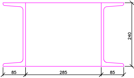
1 - horní pásnice
