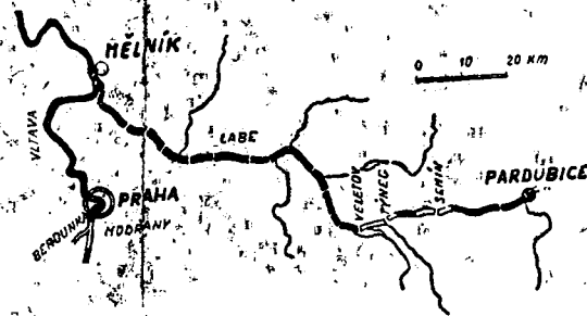
Situace splavnění středního Labe. Černé úseky jsou splavněné, bílé nejsou dosud splavněny.
