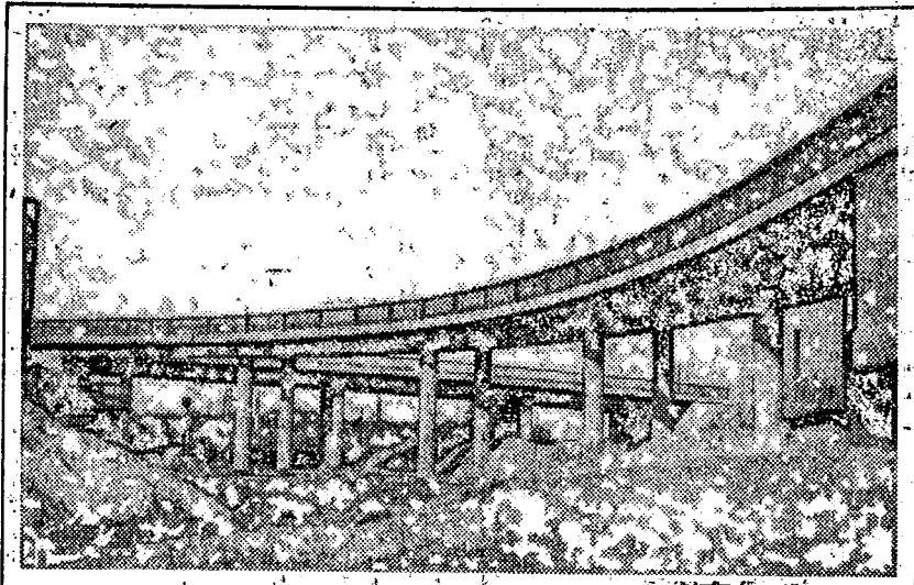
TAK TROCHU UNIKÁTNÍ bude nový nadjezd v Kolíně-Záblatí, jehož část ukazuje snímek. Po přemostění železnice se ve vzduchu na pylonech rozbíhá do dvou směrů. Tímto řešením zde budou likvidovány vlastně hned dva přejezdy, vzdálené od sebe jen několik set metrů. Foto: Miroslav Voděra
