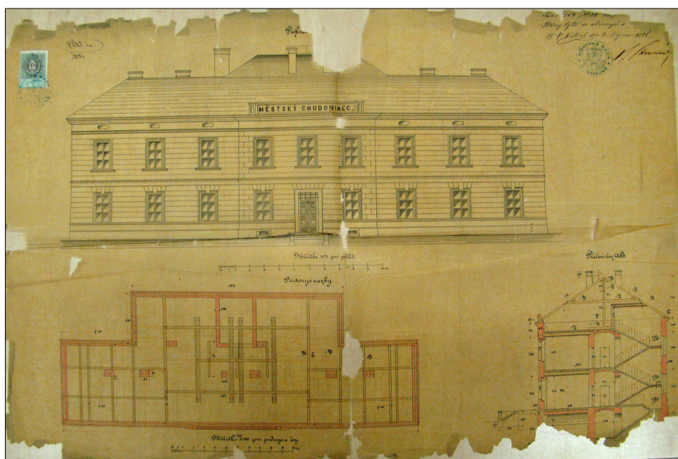
Původní projekt, dochovaný v kolínském stavebním úřadu, podle kterého byl Městský chudobinec v Kolíně v roce 1881 postaven.
