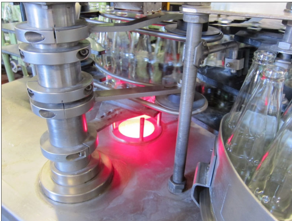
Kamerový způsob kontroly čistoty skleněných láhví s LED podsvícením
