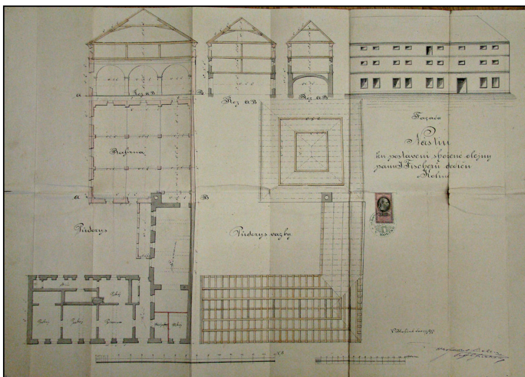
Plán na postavení šoškové olejny továrny Fischerových ze dne 27. srpna 1877
