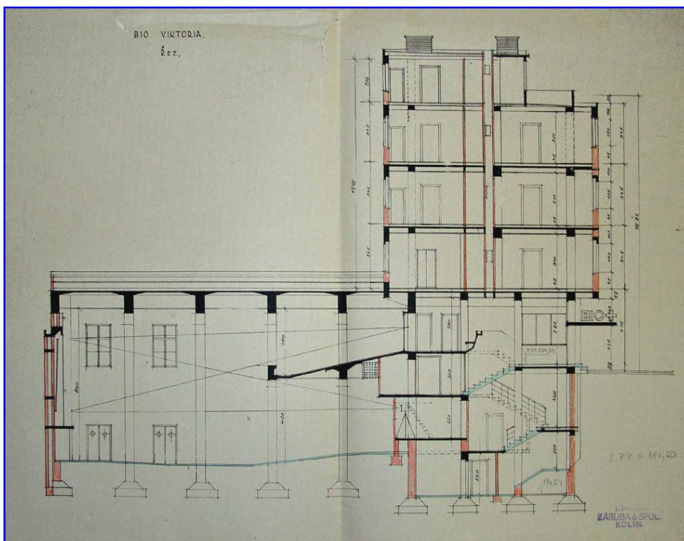
Plány na stavbu Bio Viktoria, pozdějšího kina Zálabí a konečně Jas.
