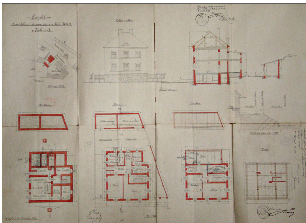
Projekt na výstavbu dezinfekční stanice ze dne 24. srpna 1924.
