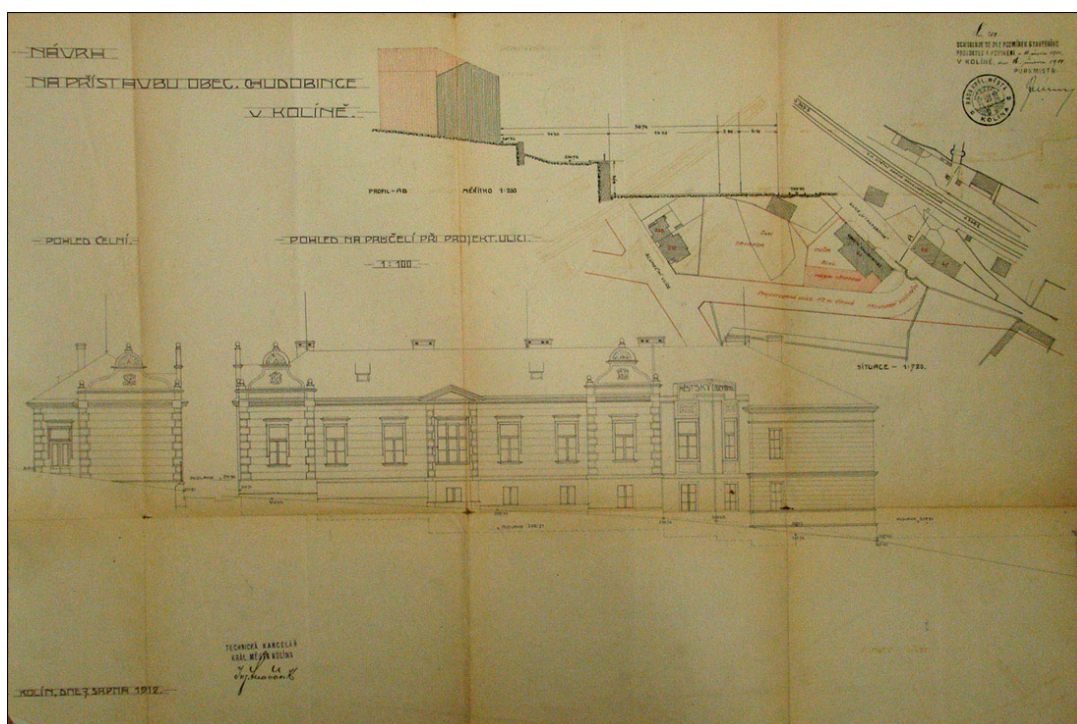
Projekt přístavby chudobince ze srpna roku 1912
