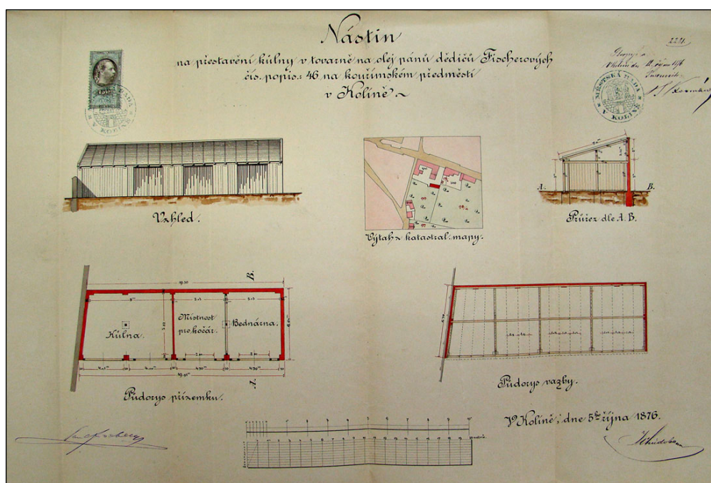
Plán na přestavbu kůlny v továrně Fischerových ze dne 5. října 1876
